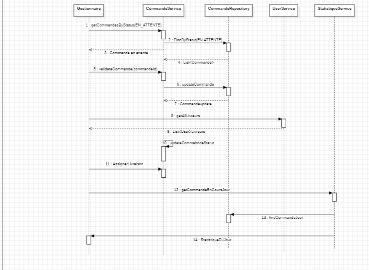
sd SequenceDiagramGestionnaire
